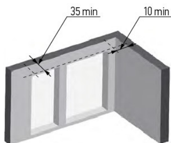
Рис. 3 Отступы до карниза
