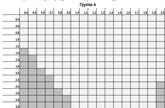
Гарантийные размеры рулонные шторы "HUNTER" труба 25 мм
