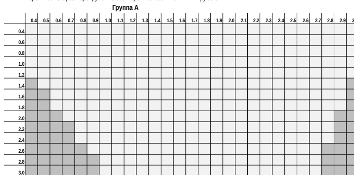
Гарантийные размеры рулонные шторы-жалюзи "HUNTER" труба 34мм
